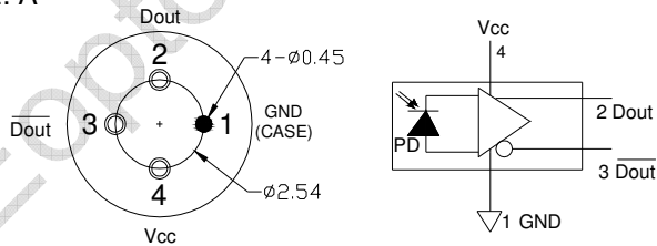
PIN-TIA-pin-A
